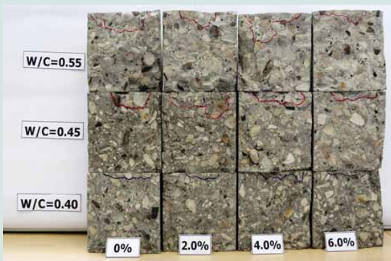
Figura 20. Efecto de Sika WT-100 sobre la penetración de agua.
