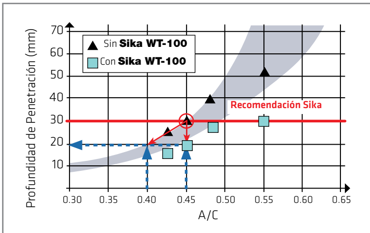
Figura 16. Resultados de Penetración de Agua vs. A/C superpuestos a resultados recientes LEM-Sika con y sin Sika WT100 [8] .
