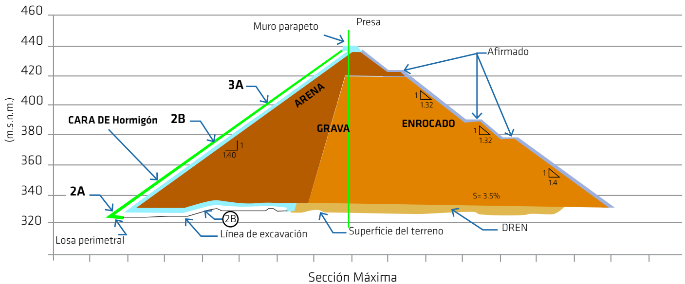
Figura 3. Esquema de una presa de enrocado y cara de hormigón (CFRD).
