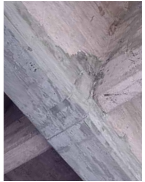
Reconstrucción de la sección mediante SikaGrout®-212 con Sikadur® 32 Gel como puente de adherencia.
